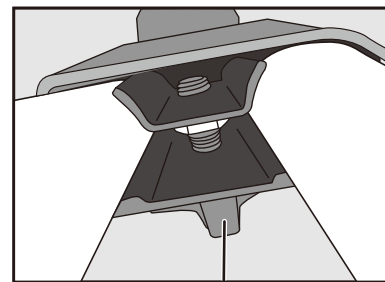
脚止めネジ
