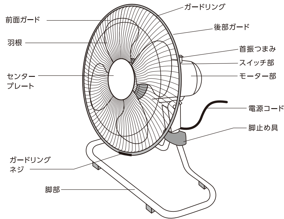
■操作パネル
