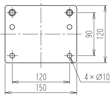
A 矢視図(取付脚穴寸法)
