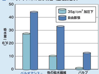
■ベルオアシス®の吸水特性 (生理食塩水)
